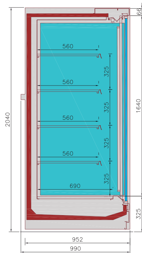
Profondeur 950
