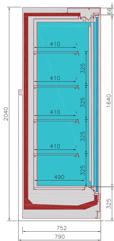
Profondeur 750
