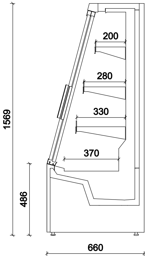
Avec portes, hauteur 1569 mm
