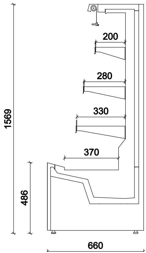
Sans porte, hauteur 1569 mm
